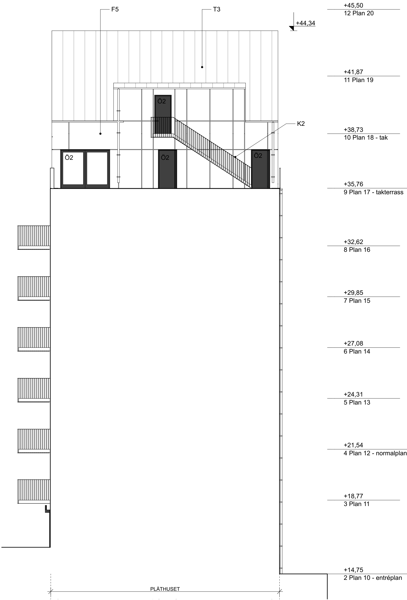
Fasad mot Sydöst 1:100
